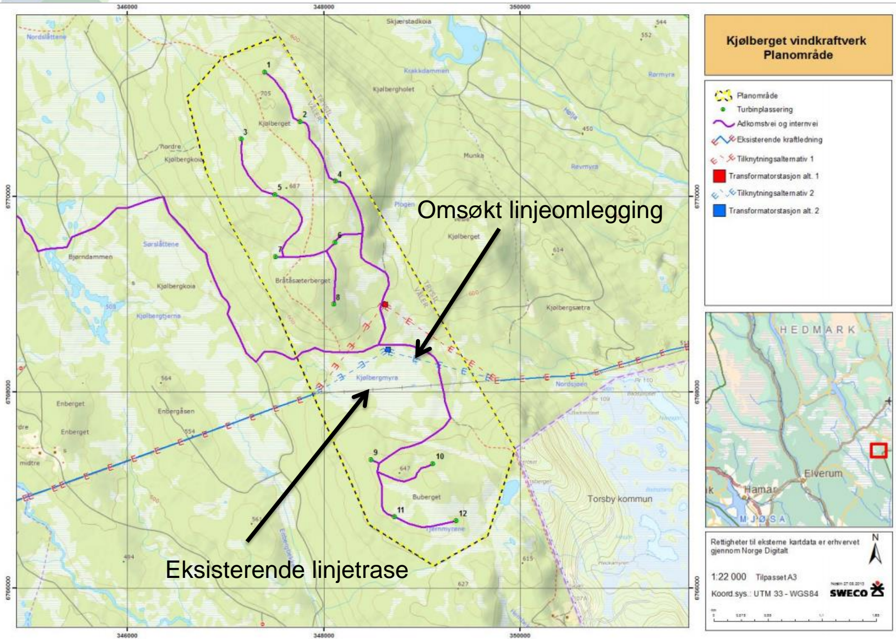
Figur 6-7 forslag til nettløsninger for Kjølerget vindkraftverk.
